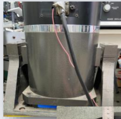
Shaker electrodinámico
